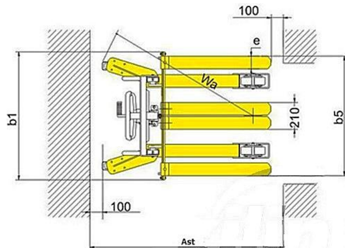
Рисунок 2. Габаритные размеры штабелера ручной SJA20E.
