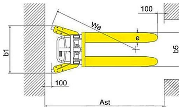
Рисунок 1. Габаритные размеры штабелера ручной SDJ.
